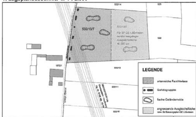
1. Lageplanausschnitt M 1 : 2.000
