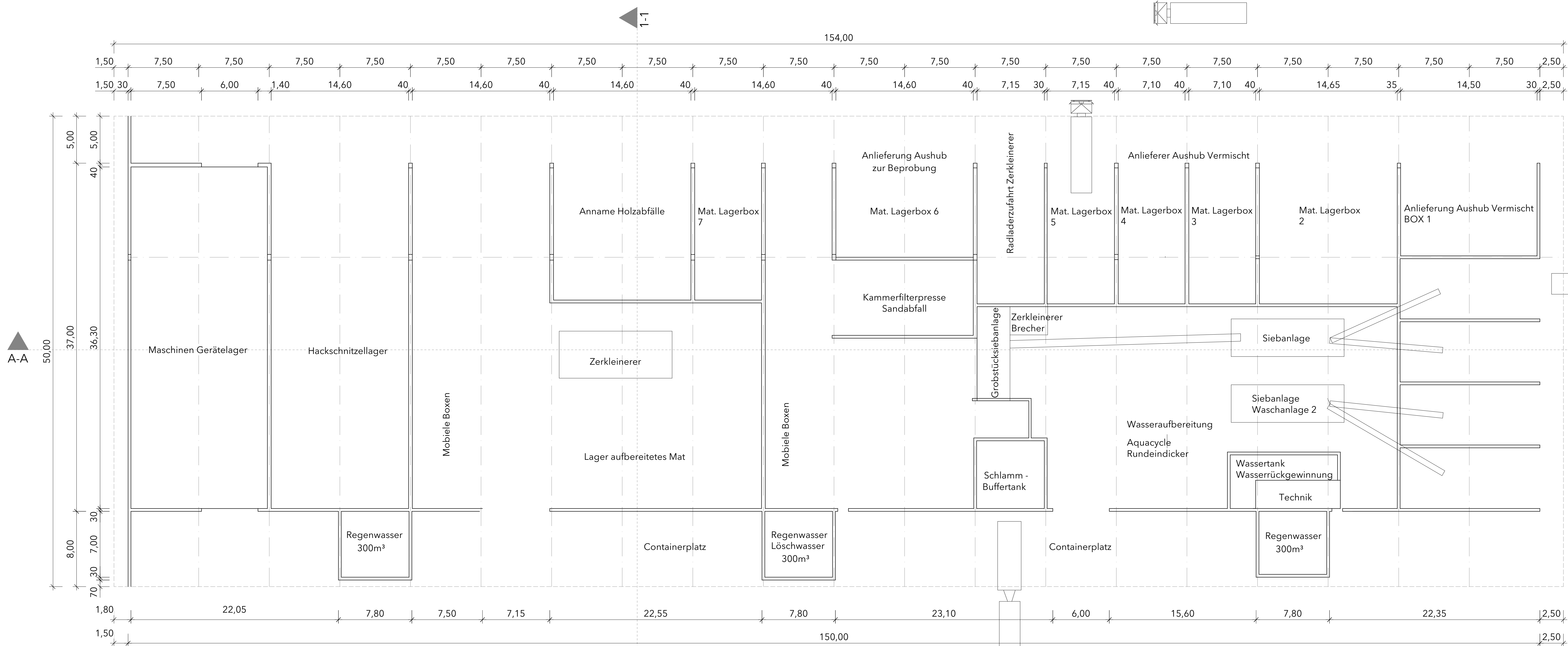
GRUNDRISS ERDGESCHOSS HALLE M 1:1.200
