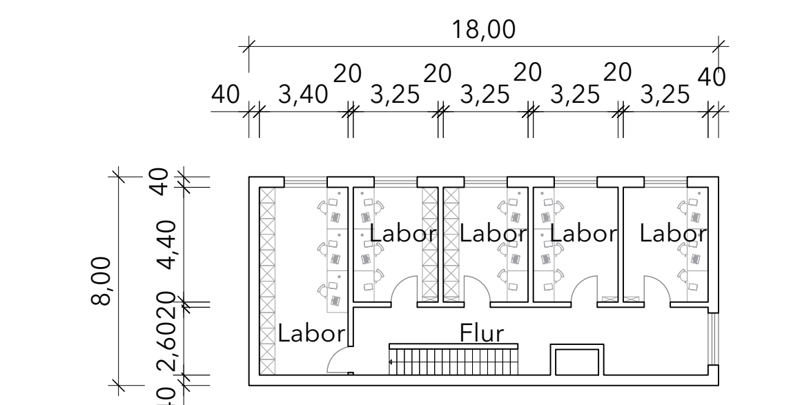
GRUNDRISS OBERGESCHOSS BÜROGEBÄUDE M 1:1.200
