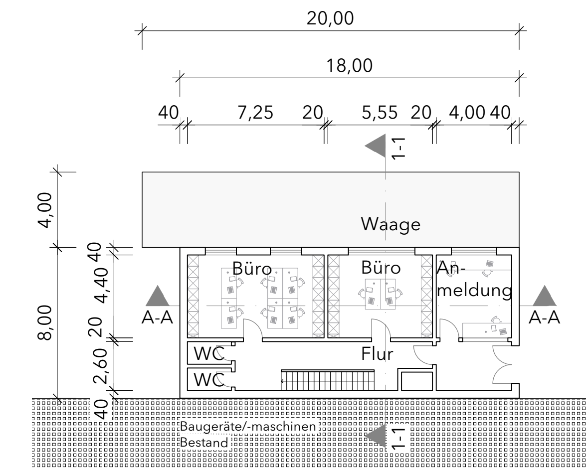
GRUNDRISS ERDGESCHOSS BÜROGEBÄUDE M 1:1.200
